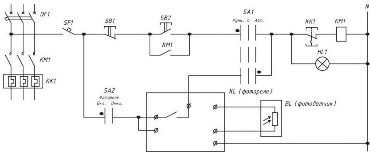
ПРИНЦИПИАЛЬНАЯ СХЕМА: ЯУ0 9602
