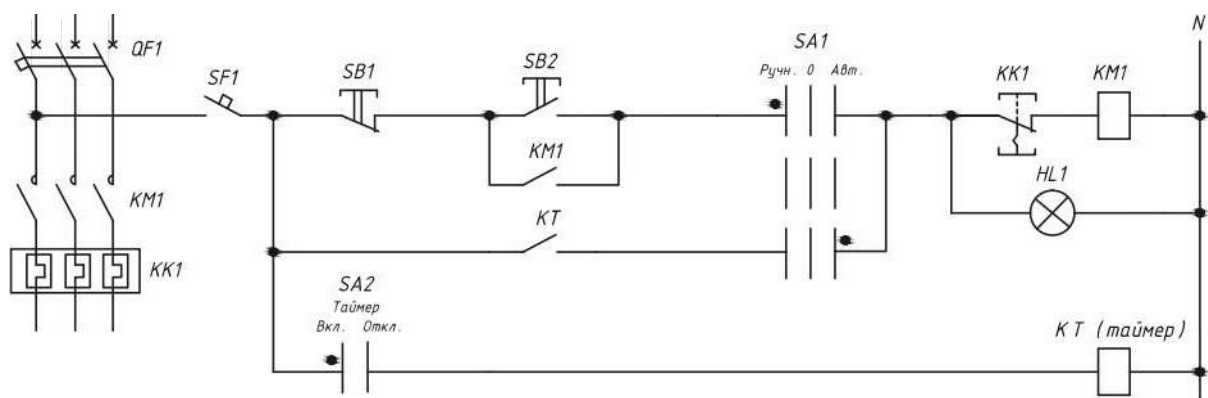
ПРИНЦИПИАЛЬНАЯ СХЕМА: ЯУ0 9603
