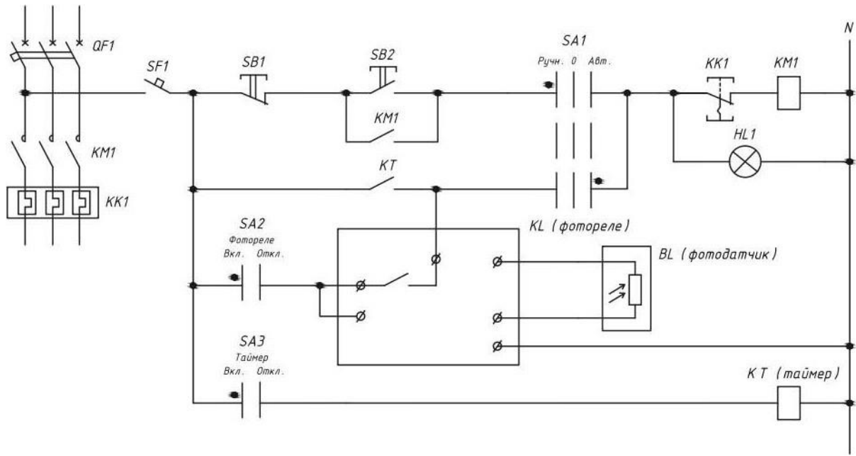
ПРИНЦИПИАЛЬНАЯ СХЕМА: ЯУ0 9601
